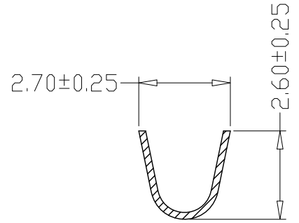
SEC: A-A
