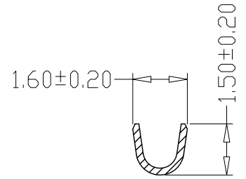
SEC: B-B
